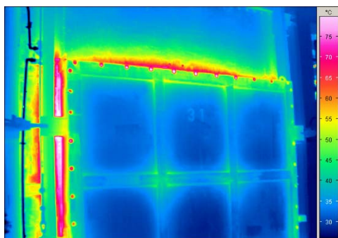
Brennofentür
