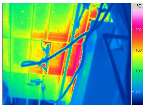
Aluminiumofen
